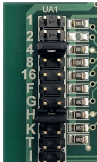
Bild utvisande bygel H och 4 är på. (Betyder fristående drift och endast spjällgrupp 1 används.)
